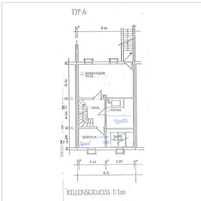
Grundriss_KG
